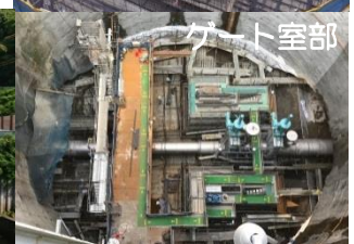
減勢池部
